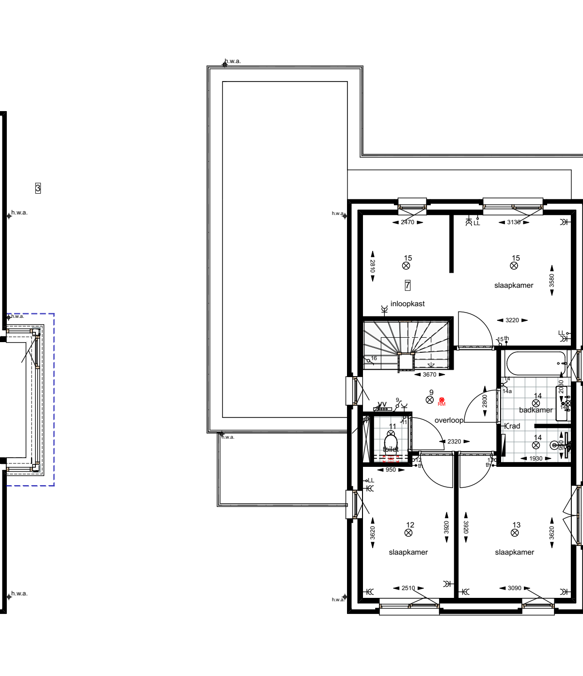
1e verdieping Optie 7 Bouwnummer(s): 1.13 Bouwnummer(s): 1.26 gespiegeld
