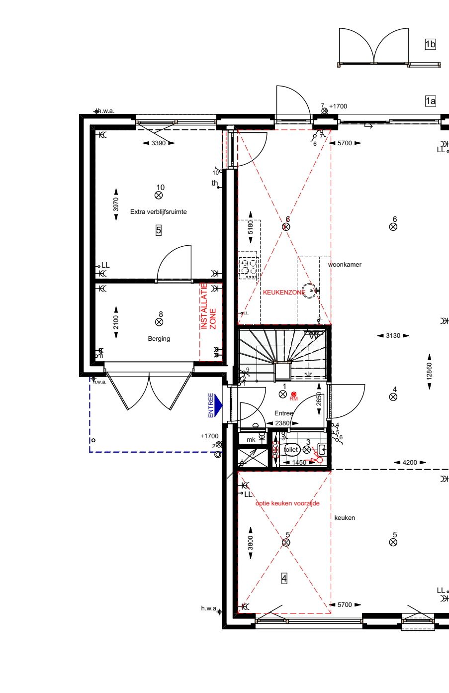
Begane grond Opties 1a+1b+3+4+5 Bouwnummer(s): 1.13
