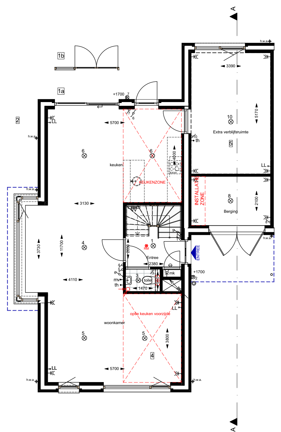
Begane grond Opties 1a+1b+2+4+5+6+10 Bouwnummer(s): 1.26
