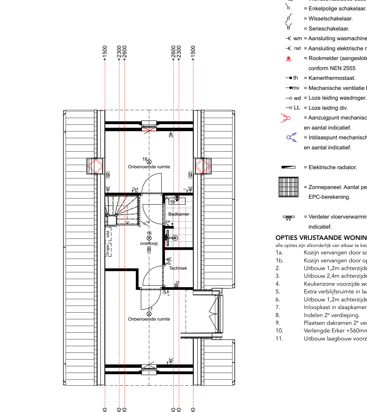
2e verdieping Optie 8+9 Bouwnummer(s): 1.13 Bouwnummer(s): 1.26 gespiegeld
