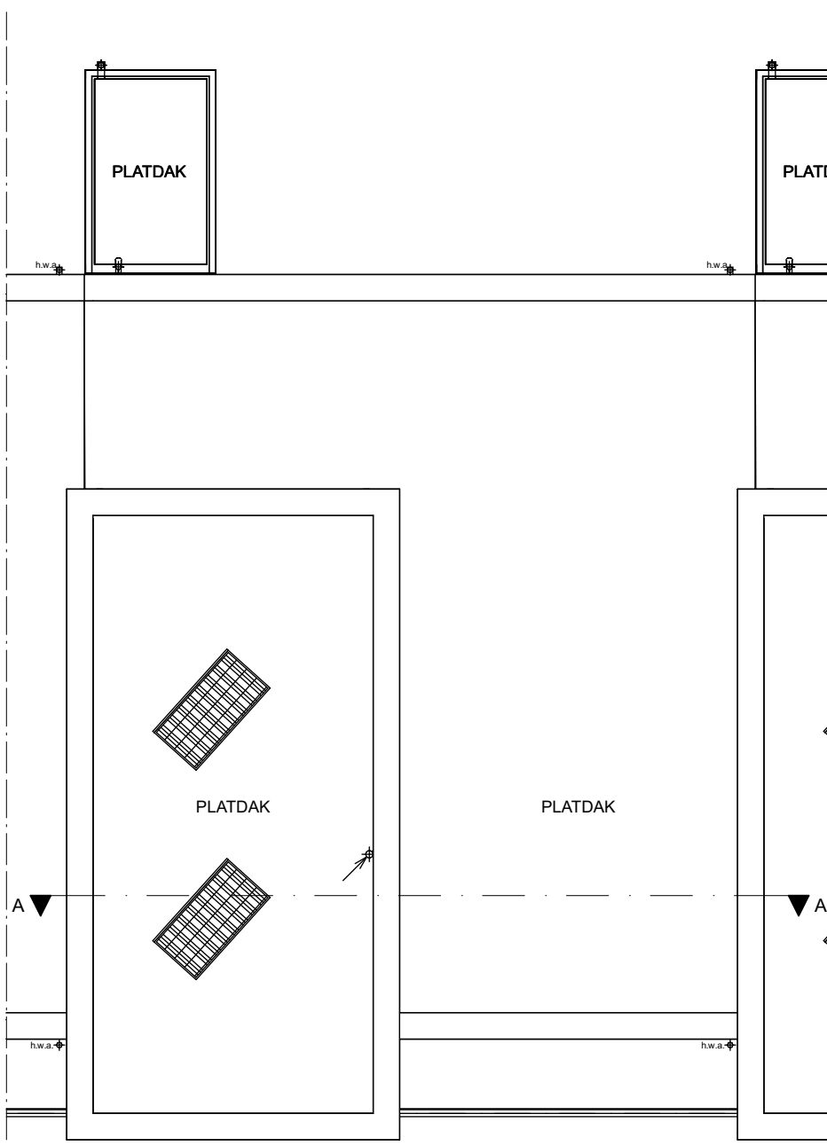
Dakaanzicht Bouwnummer(s): 1.07 t/m 1.12. Bouwnummers 1.07 en 1.12 voorzien van eindgevel.
