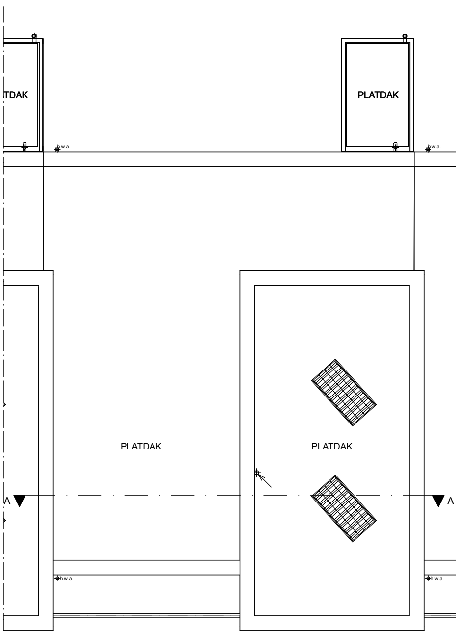
Dakaanzicht Bouwnummer(s): 1.02 t/m 1.06. Bouwnummer 1.06 voorzien van eindgevel.
