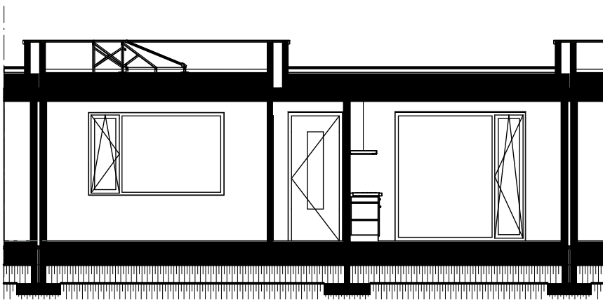
Doorsnede A-A Bouwnummer(s): 1.02 t/m 1.06. Bouwnummer 1.06 voorzien van eindgevel.
