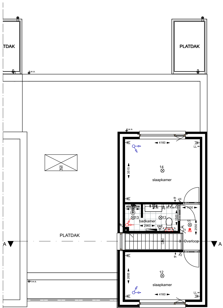
1e verdieping optie 4
