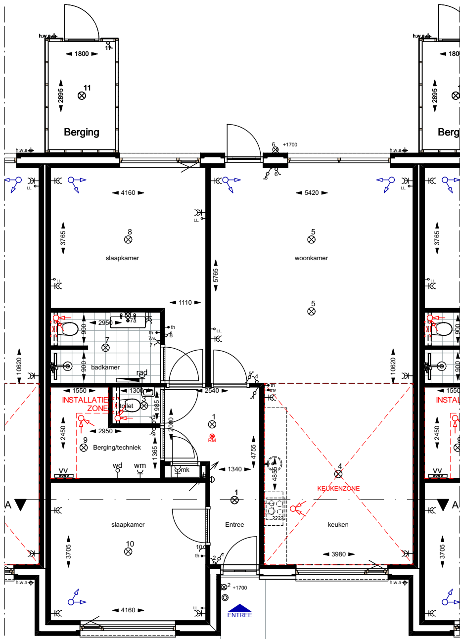
Begane grond Bouwnummer(s): 1.07 t/m 1.12. Bouwnummers 1.07 en 1.12 voorzien van eindgevel.
