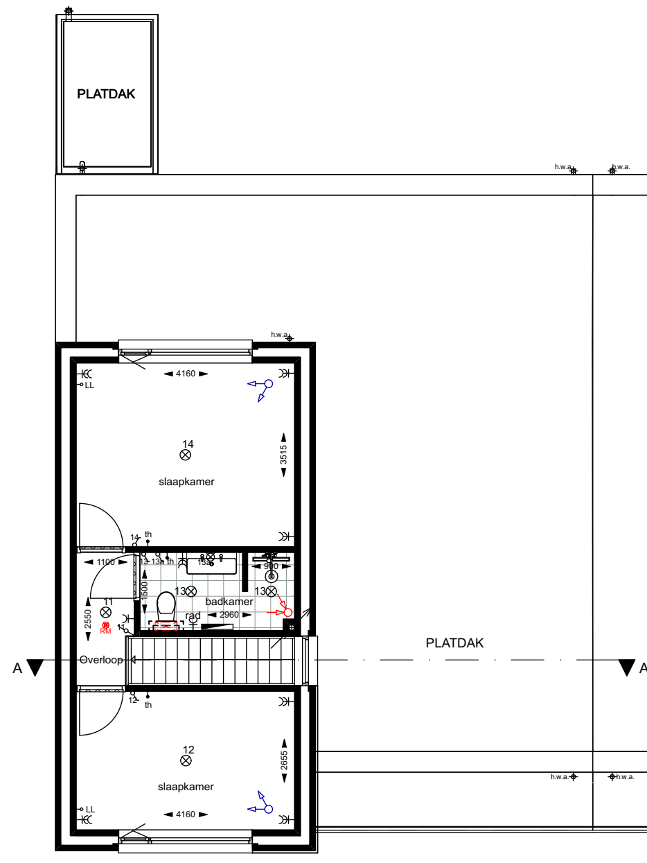
1e verdieping Bouwnummer(s): 1.01
