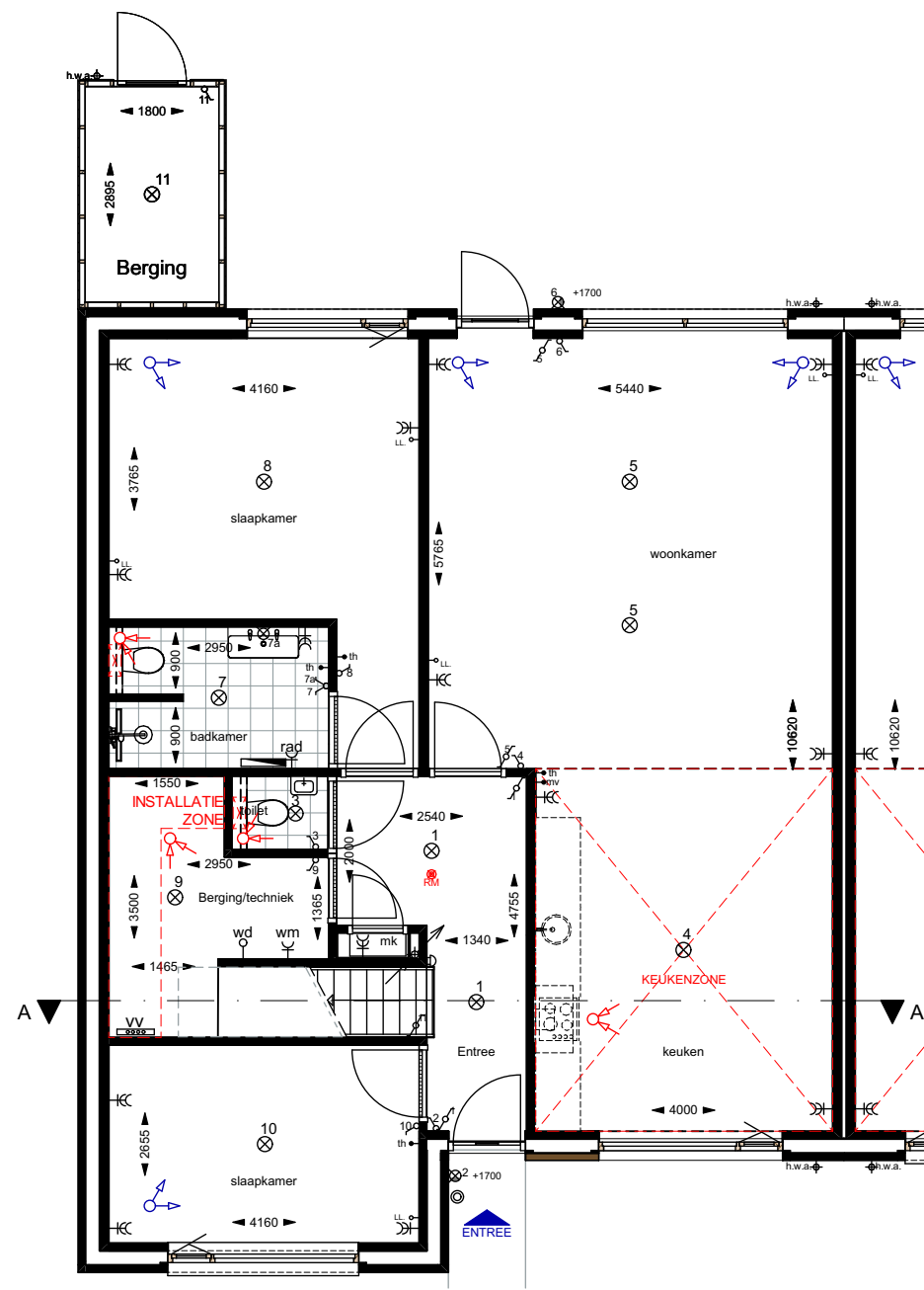
Begane grond Bouwnummer(s): 1.01
