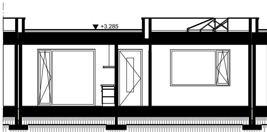
Doorsnede A-A Bouwnummer(s): 1.07 t/m 1.12. Bouwnummers 1.07 en 1.12 voorzien van eindgevel.
