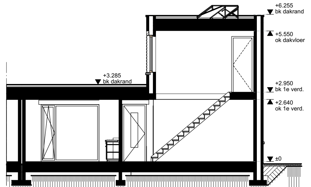
Doorsnede A-A Bouwnummer(s): 1.01
