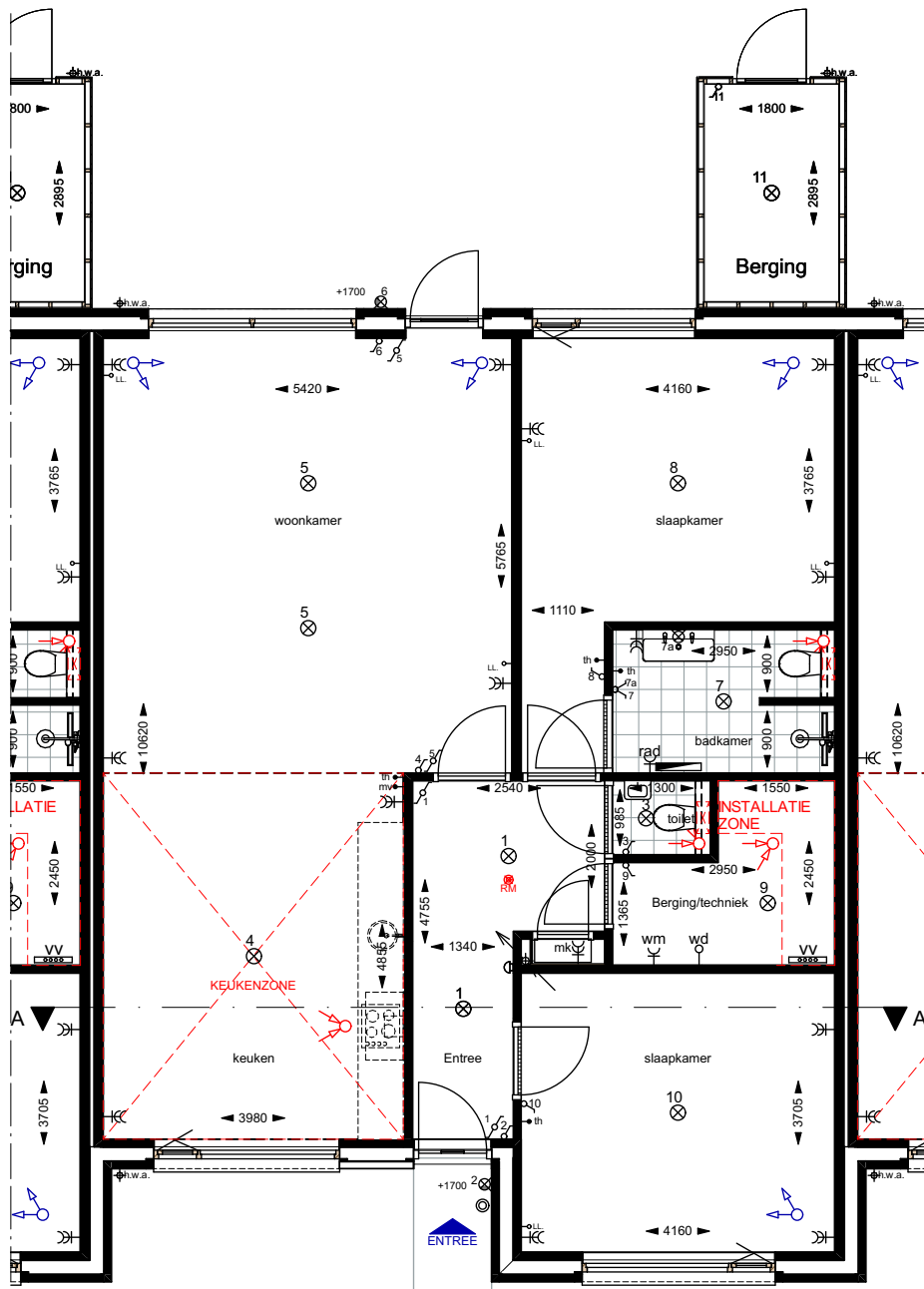
Begane grond Bouwnummer(s): 1.02 t/m 1.06. Bouwnummer 1.06 voorzien van eindgevel.
