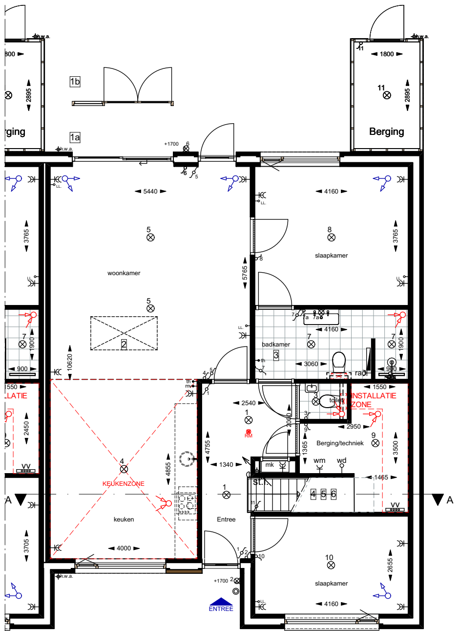
Begane grond optie 4+5+6
