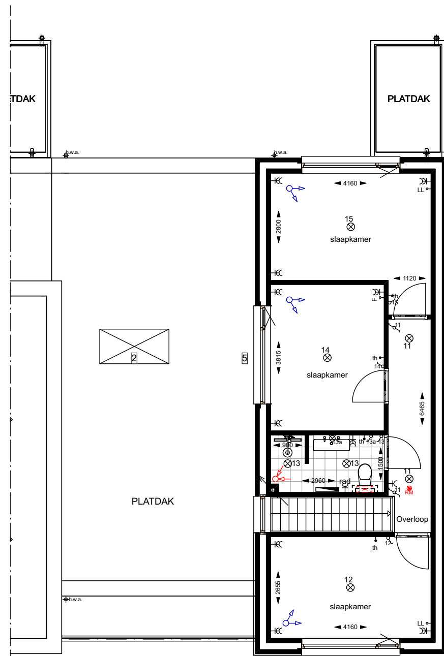
1e verdieping optie 5
